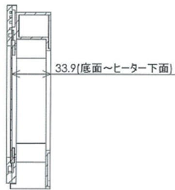
断面図 A-A
